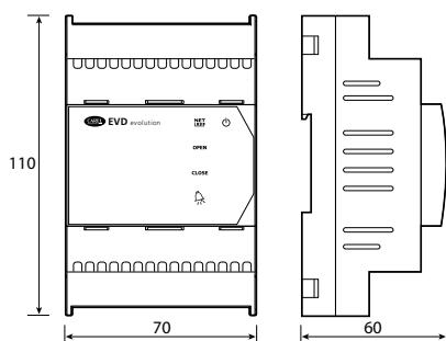
Габаритные размеры, мм
