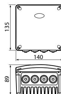
Габаритные размеры, мм
