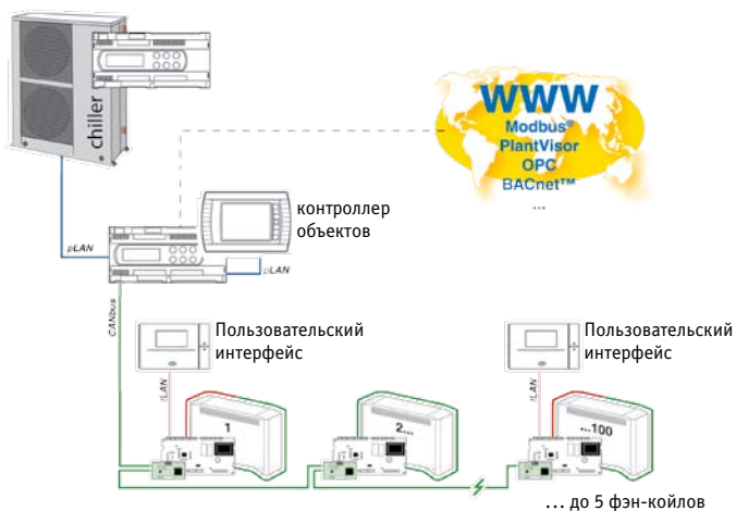
multimaster e-drobus
