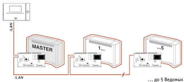
Передача в стандартном диапазоне
