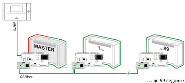
Передача в расширенном диапазоне
