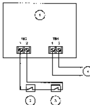
Рисунок 18 - Подключение термостата пожарной сигнализации к плате ТС1
